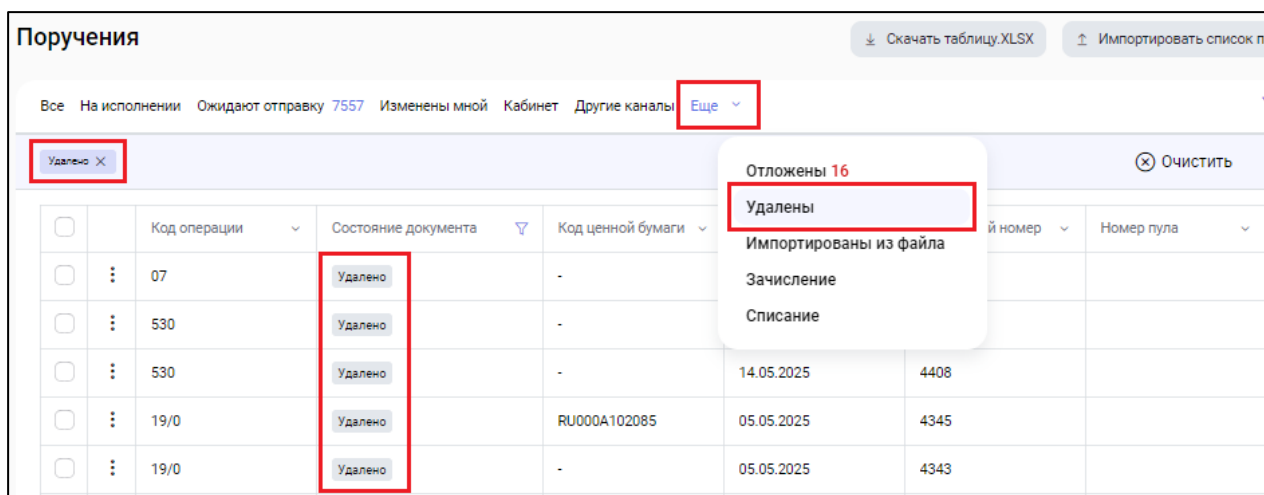
Рисунок 153 Фильтр «Удалены»
