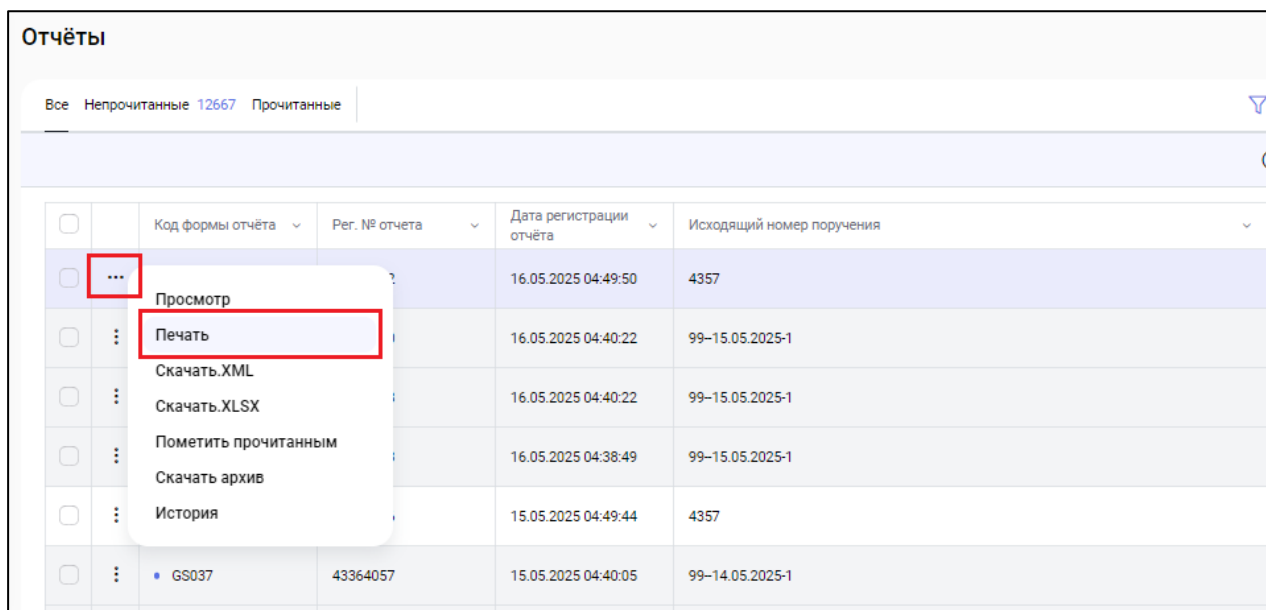
Рисунок 224 Печать отчета
