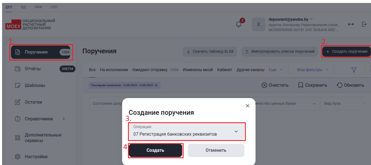
Рисунок 118 Создание 07 поручения
