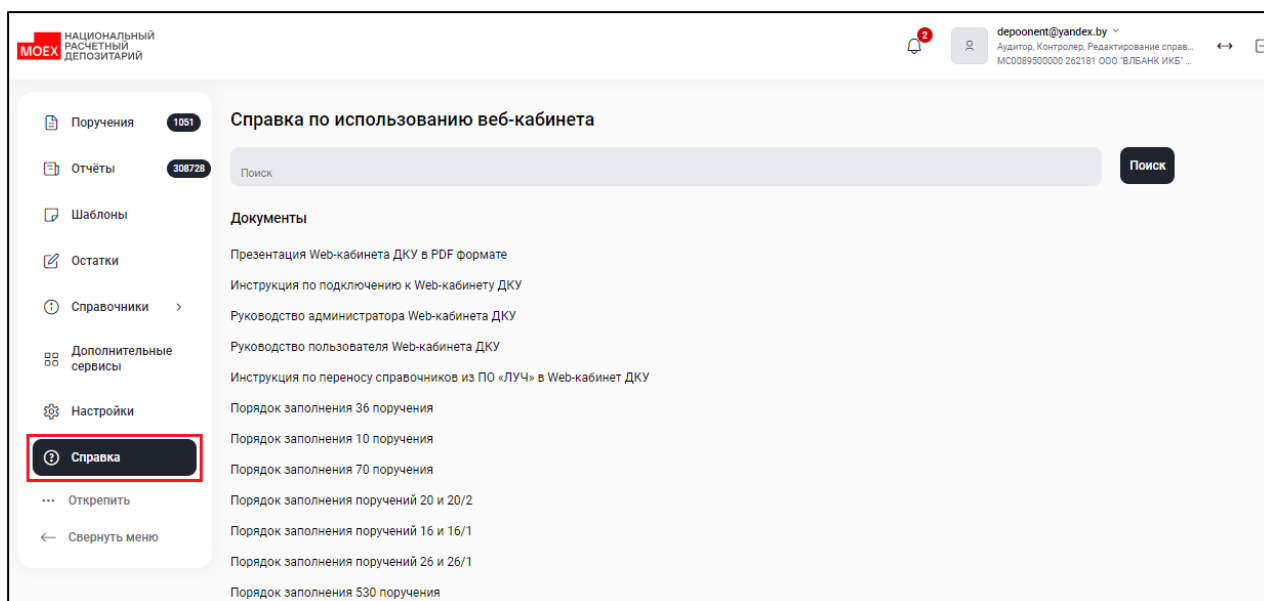
Рисунок 283 Раздел «Справка»
