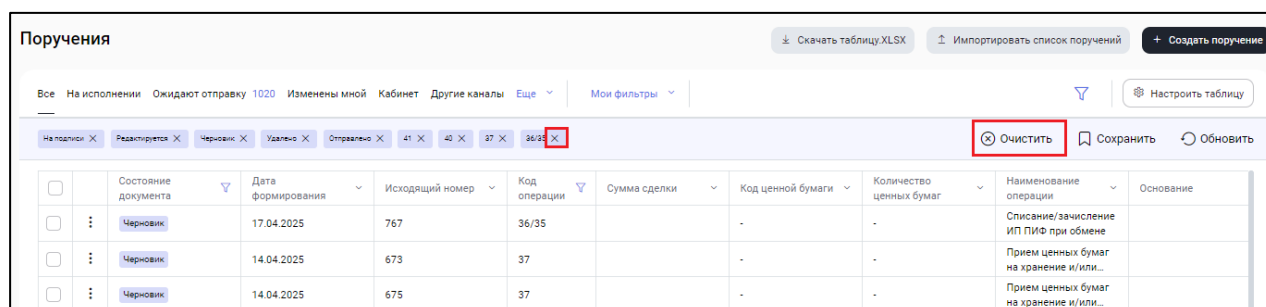
Рисунок 34 Удаление фильтров
