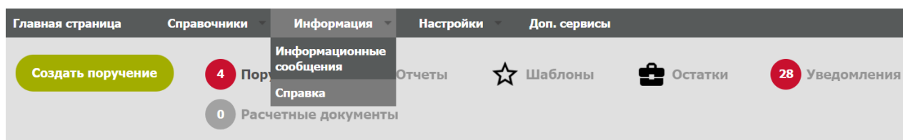
Рис. 176 Подраздел "Справка"
