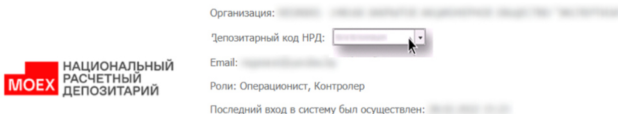
Рис. 1 Выбор организации
