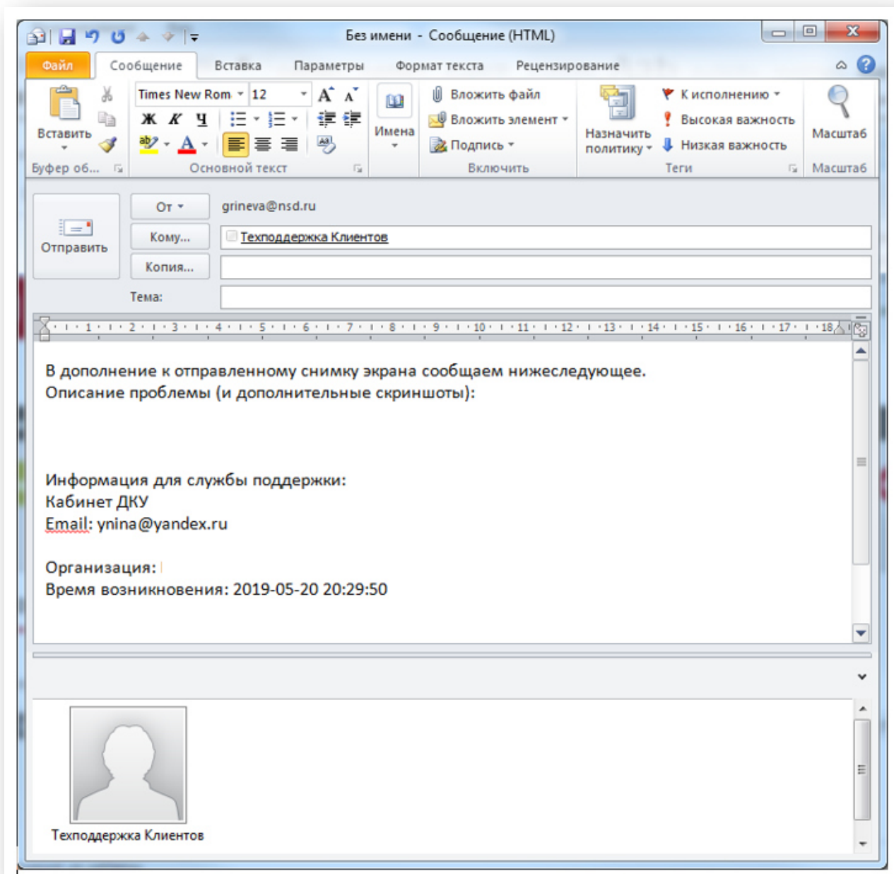
Рис. 193. Сопроводительное письмо
