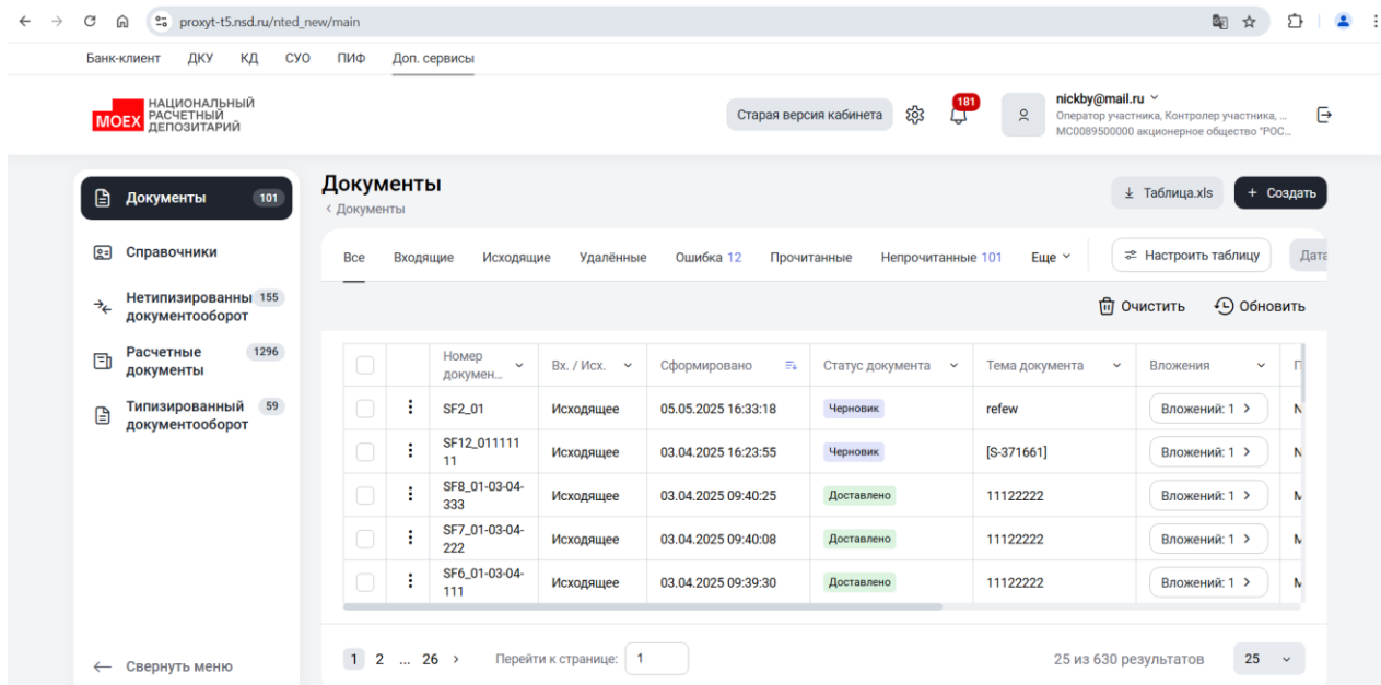
Рисунок 3 Главная страница
