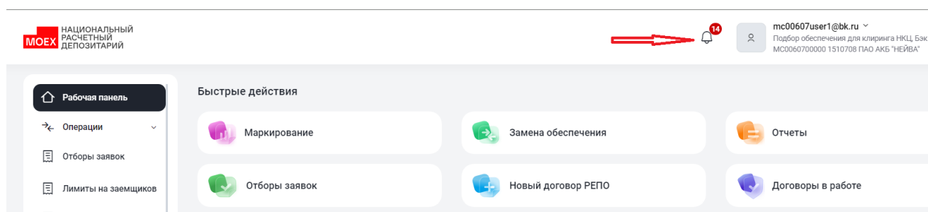
Уведомление
