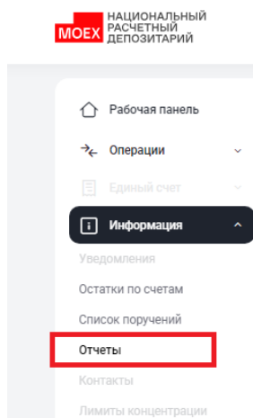
Меню "Отчеты"
